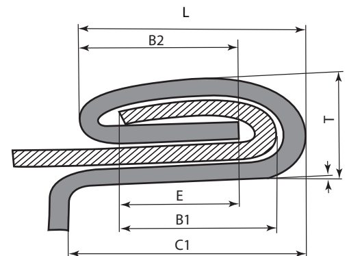
Схема закаточно шва / Scheme of seam
