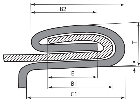
Схема закаточного шва / Scheme of seam
