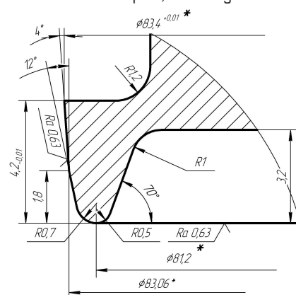
закаточный патрон / seaming chuck
